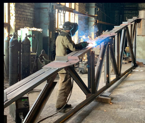
Изготовление фермы
